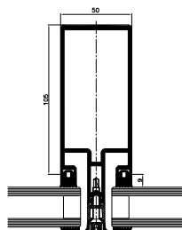
przekrój przez słup
