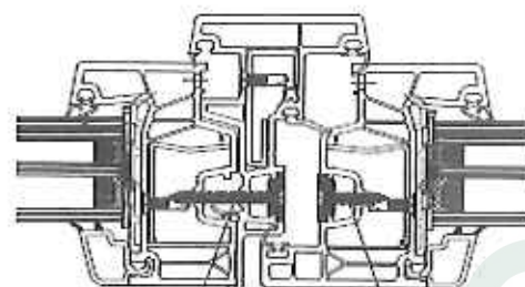
Beschlagschraube 3,9x40
