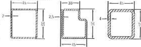
Pfosten 124 AD/MD
