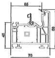
9003 .. Blendrahmen 70/78 5K
