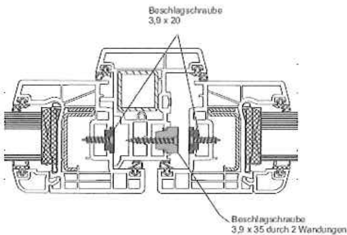
Beschlagsausführung "Stulp mit 2. Griffolive"
