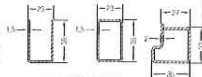
Pfosten 124 AD/MD
