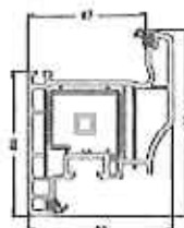
8 648 .. Flügelrahmen 82/103 4K
