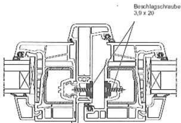
Beschlagsausführung "Stulp mit Stulpgetriebe GASM/GASK"
