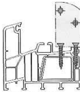
Kömmerling 88+ Bauteilserie 144
