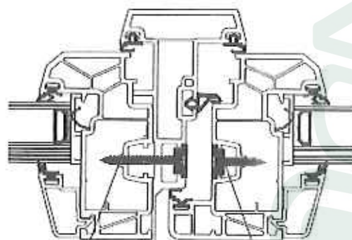
Beschlagschraube 3,9x40
