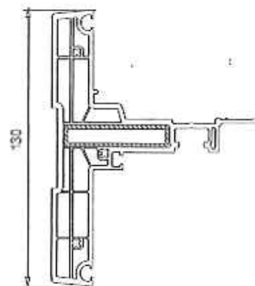
Stützprofil 102.325 Stahl 113.013
