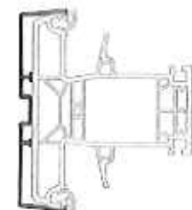
Vorsatzschale für Pfosten 06 AD/MD
