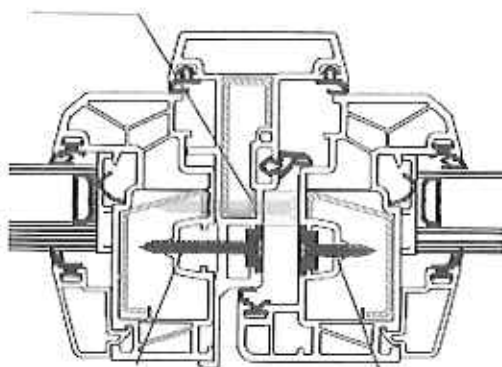
Beschlagschraube 4,1 x40
