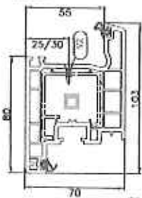
Flügelrahmen 70/103 3K 8563..
