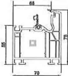
9006 .. T-Prof 70/91 3K
