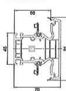
9007 .. T-Prof 70/91 5K
