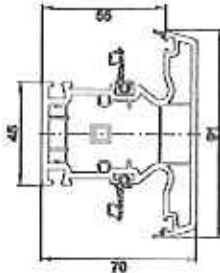
9006 .. T-Prof 70/91 3K
