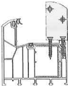
KBE 88+ Bauteilserie 205
