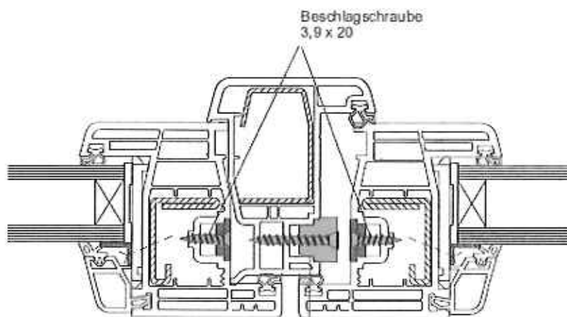
Beschlagsausführung "Stulp mit 2. Griffolive"
